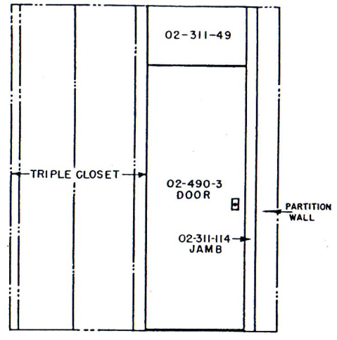
(24) ELEVATION INSIDE BEDROOM N° 2
